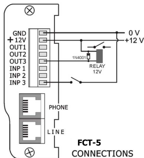
Σχήμα 1: Συνδέσεις του FCT-5 SMS
